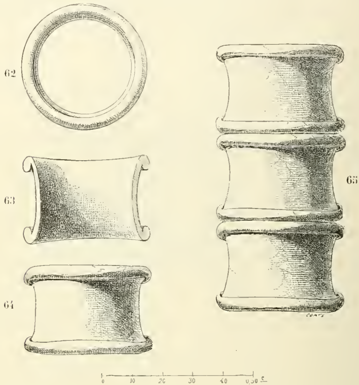
62. — Manchon de terre cuite, plan. Place, Ninive , t. III, pl. 67.
